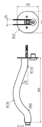
Modèle présenté AD25501- 300 mm Finition 000. Supermirror
