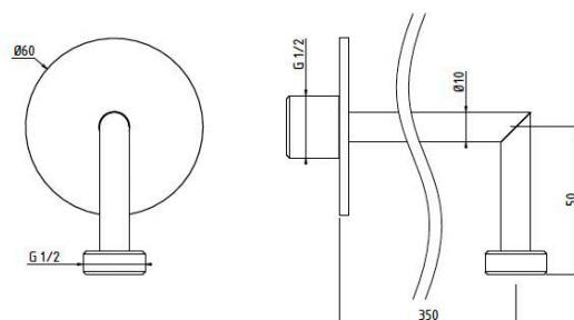
Modèle présenté AD25235 - 350 mm Finition 000. Supermirror
