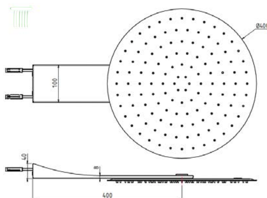
Modèle présenté AD34533 Finition 000. Supermirror
