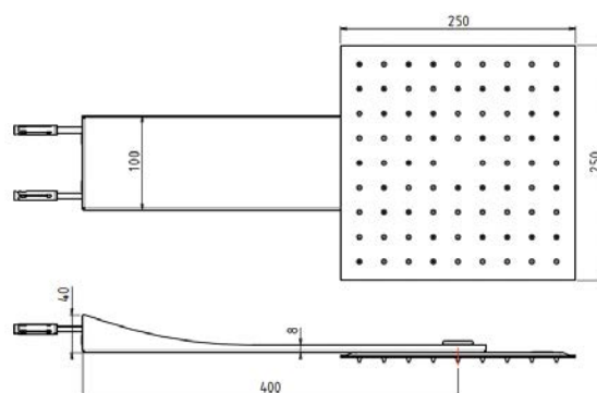
Modèle présenté AD34613 Finition 000. Supermirror
