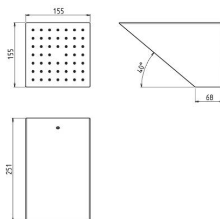
Modèle présenté AD5125 Finition 000. Supermirror
