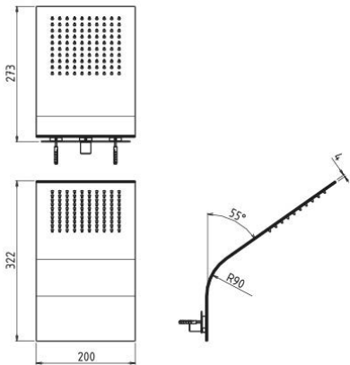
Modèle présenté AD35031 Finition 000. Supermirror
