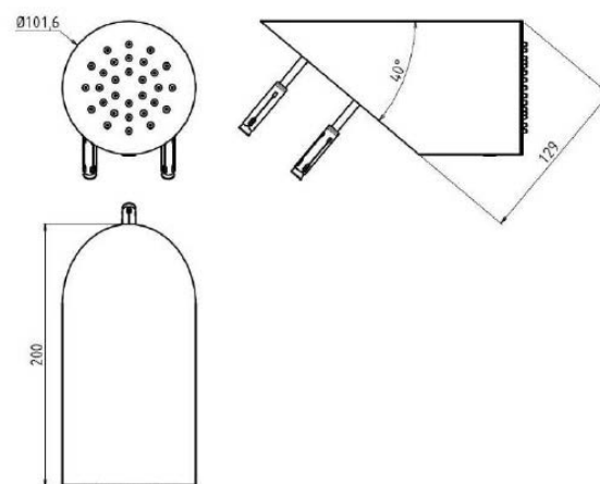
Modèle présenté AD5116 Finition 000. Supermirror
