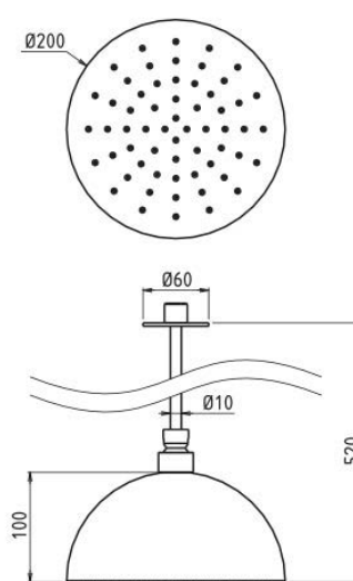
Modèle présenté AD36002 Finition 000. Supermirror
