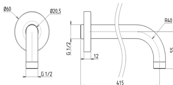
Modèle présenté AD25632 - 400 mm Finition 000. Supermirror
