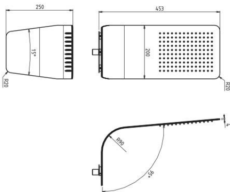
Modèle présenté AD35030 Finition 000. Supermirror
