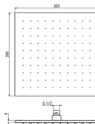
Modèle présenté AD39313 Finition 000. Supermirror
