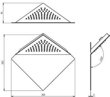
Modèle présenté AD35035 Finition 000. Supermirror
