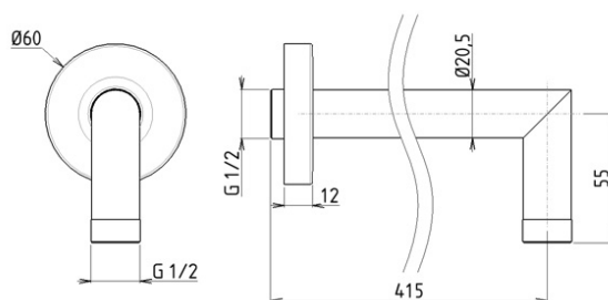
Modèle présenté AD25297 - 400 mm Finition 000. Supermirror
