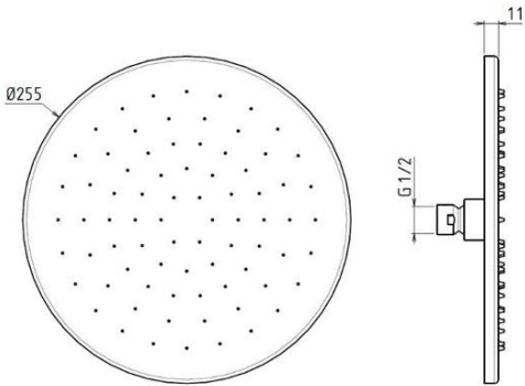
Modèle présenté AD39400 Finition 200. Supermirror Longlife
