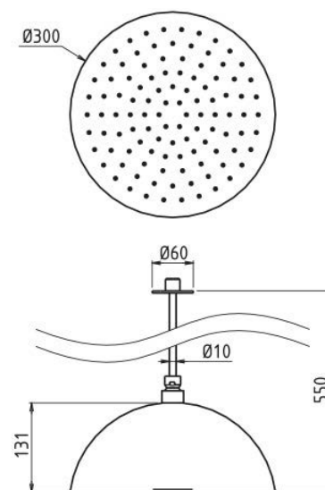
Modèle présenté AD36012 Finition 000. Supermirror
