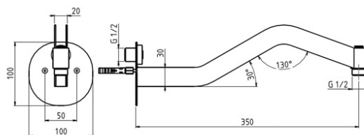
Modèle présenté AD25500 - 350 mm Finition 000. Supermirror
