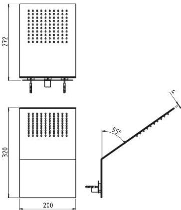
Modèle présenté AD35032 Finition 000. Supermirror
