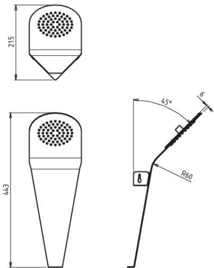
Modèle présenté AD35050 Finition 000. Supermirror
