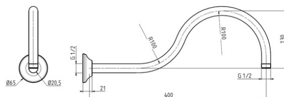
Modèle présenté AD25540 - 400 mm Finition 000. Supermirror
