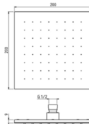
Modèle présenté AD39311 000. Supermirror
