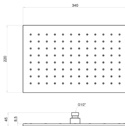
Modèle présenté AD39320 Finition 000. Supermirror
