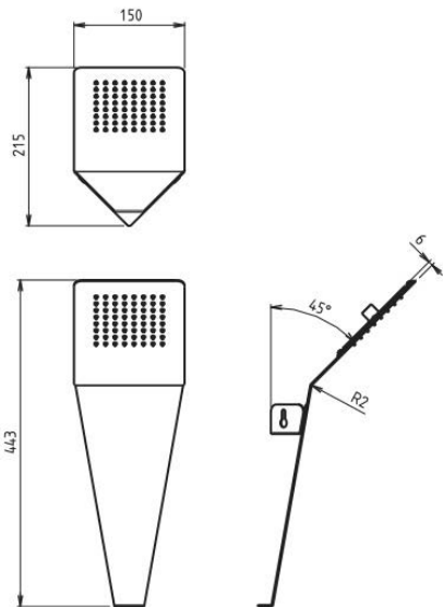
Modèle présenté AD35040 Finition 000. Supermirror
